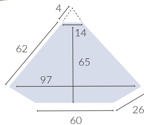
Modelo 612 Rinconera tv ↑ 80 ↔ 98 ↗ 62 cm Puntos: Pulimento 277 / Lacado: 329
